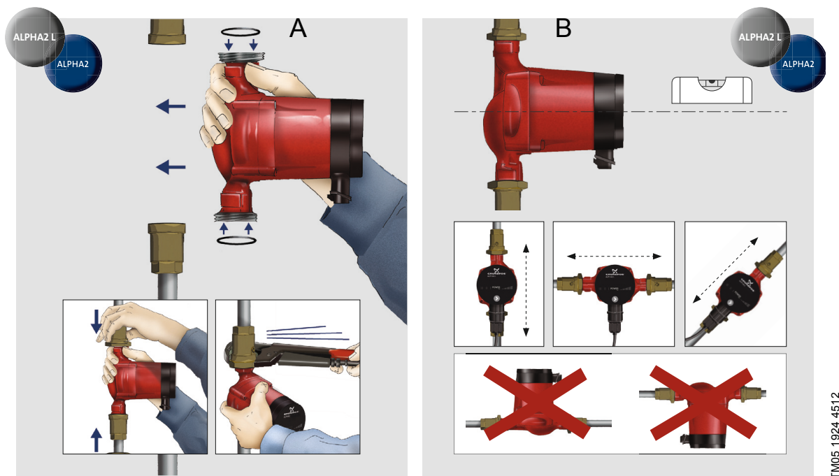
Fig. 3 Montering av GRUNDFOS ALPHA2 L
