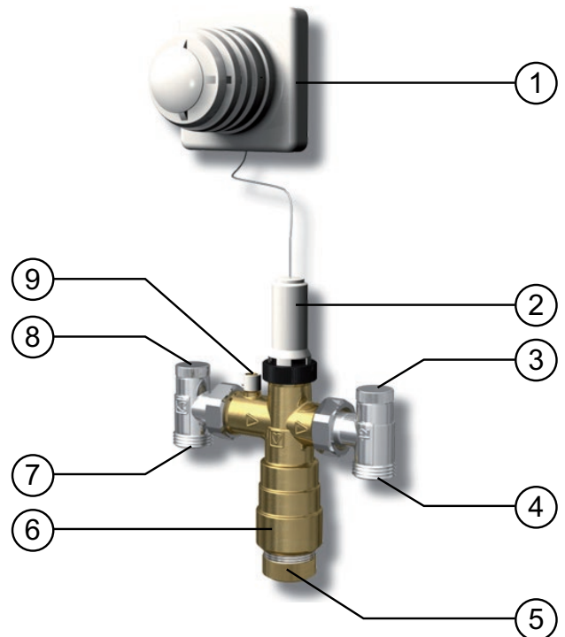
LK Minikretsventil M5.
