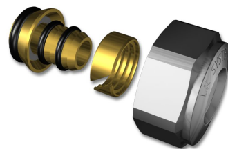
LK Anslutningskoppling RF.
