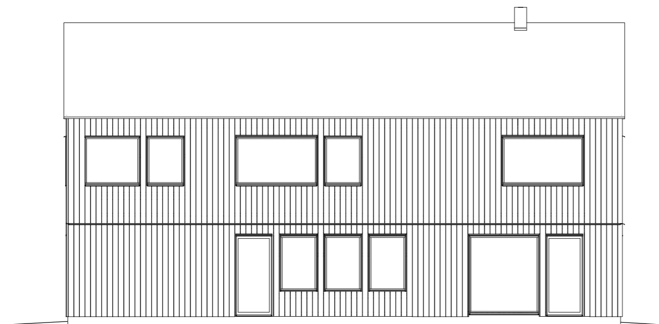
FASAD SÖDER
