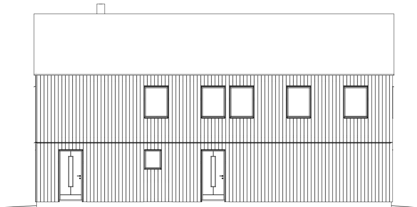
FASAD NORR
