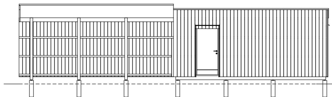
FASAD SÖDER
