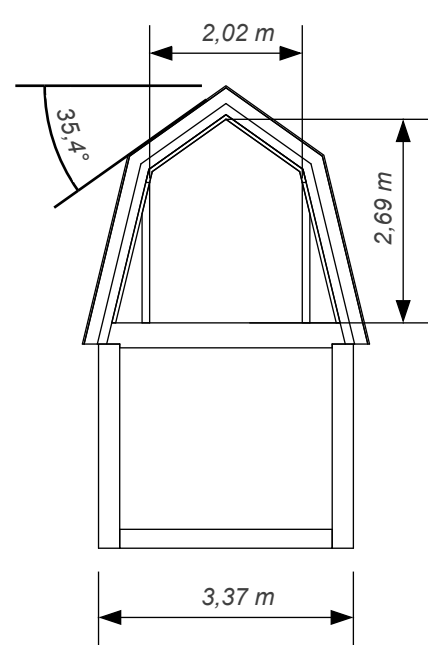
Sektion A-A
