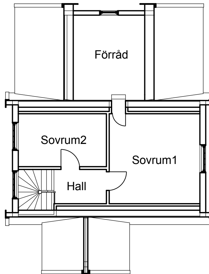
Befintligt Plan 2
