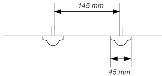
Sektion Fasadbeklädnad, hattläkt Skala 1:5
