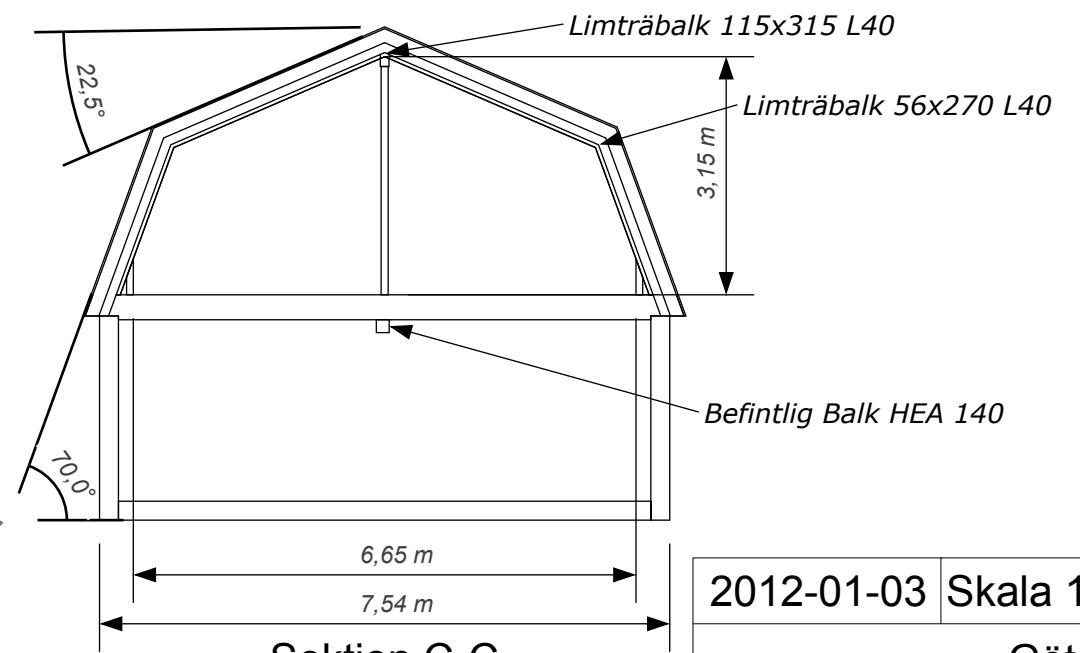
Sektion C-C
