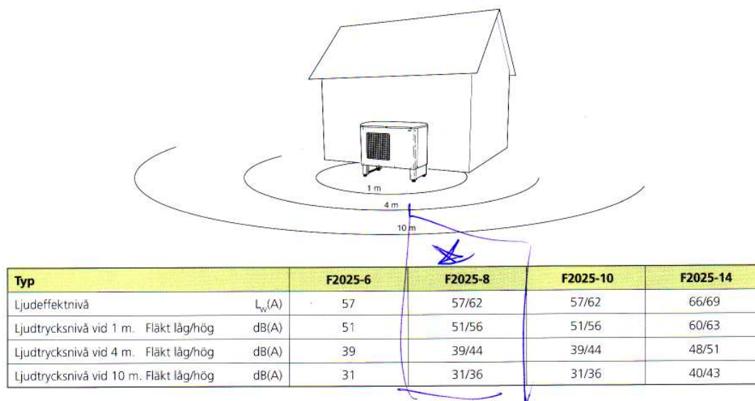
Figur 1. Tabell från informationsbroschyr Nibe F2025
