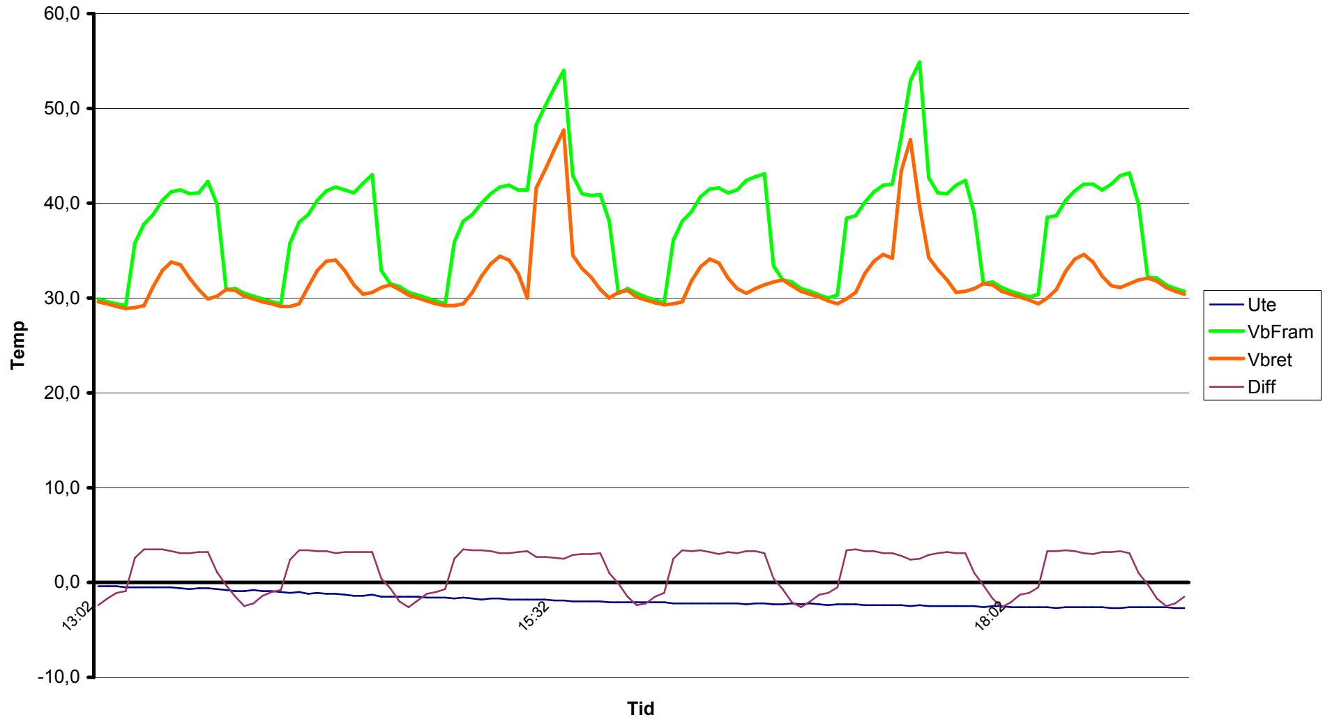
1245-10 Radiator 240 kvm + golvvärme 60 kvm Stockholm. Kurva=8 Period: 16-17 Dec
