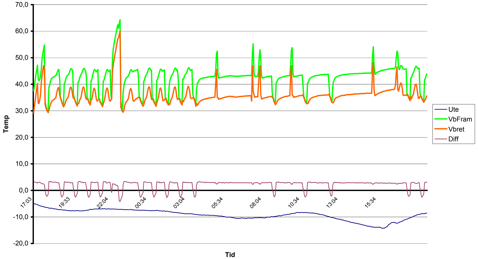
1245-10 Radiator 240 kvm + golvvärme 60 kvm Stockholm. Kurva=8 Period: 14-15 Dec
