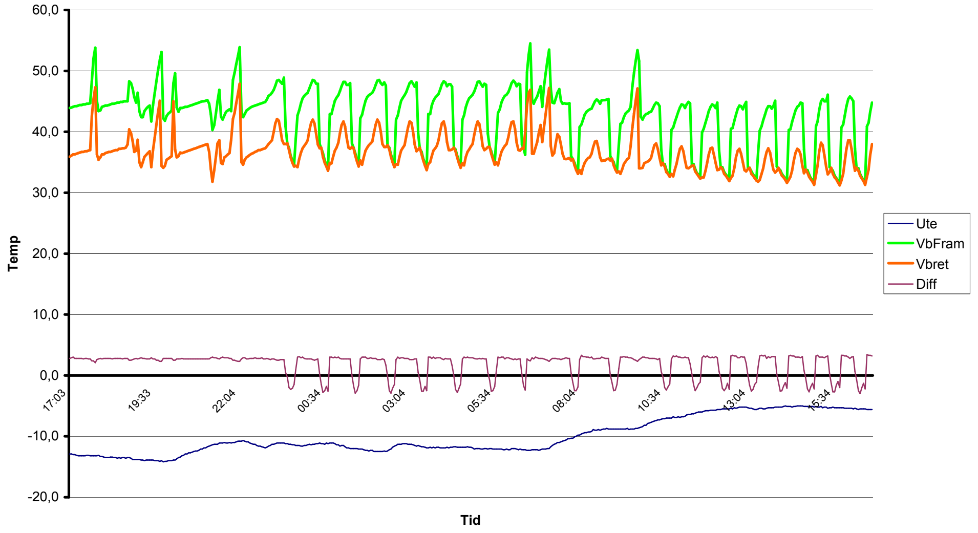
1245-10 Radiator 240 kvm + golvvärme 60 kvm Stockholm. Kurva=8 Period: 12-13 Dec
