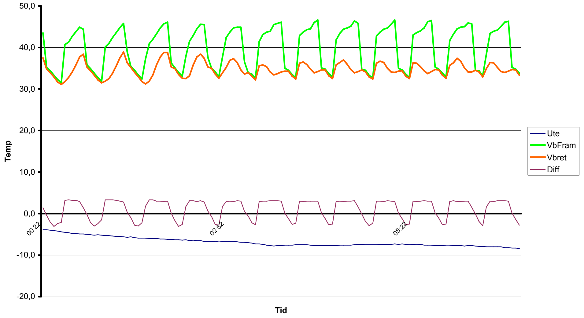
1245-10 Radiator 240 kvm + golvvärme 60 kvm Stockholm. Kurva=8 Period: 11-12 Dec
