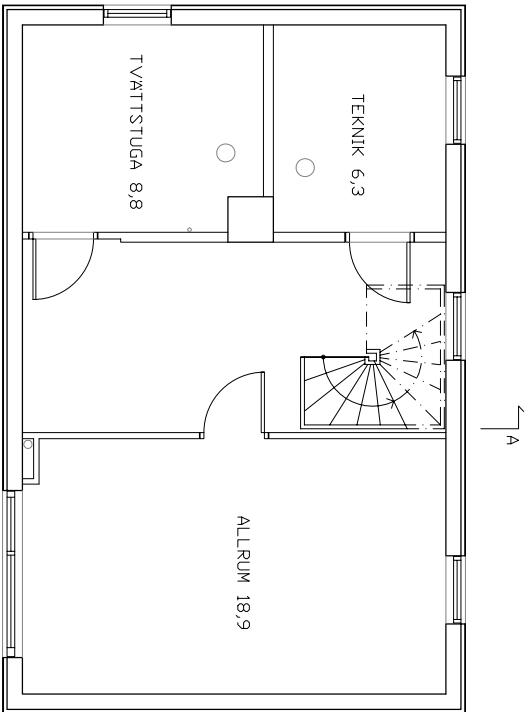
Källarplan
