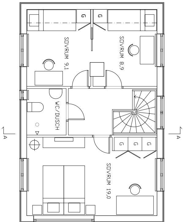
Övre plan
