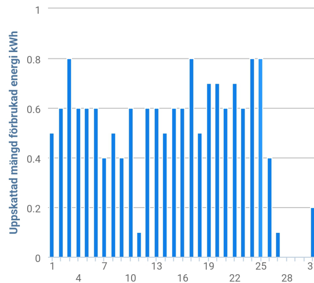
Uppskattad mängd förbrukad energi Mitsubishi AP-25: 01/07/2021 - 31/07/2021
